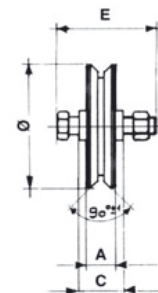
Kotač
