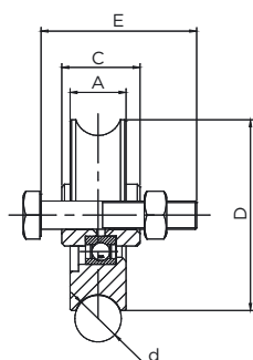
Kotač
