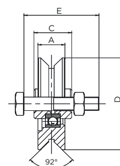
Kotač
